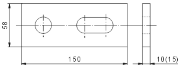
■ 中間圈用卡具 Plate for Center Gland (CNS 2473之SS 400或尼龍6) (SS 400 or nylon 6 of CNS 2473)
