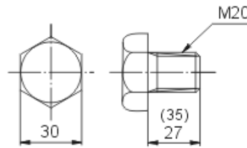
■ 中間圈用卡具用螺栓 Bolts for Plate (CNS 2473之SS400或 CNS 3270之304) (SS 400 of CNS 2473 or 304 of CNS 3270)
