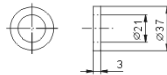
■ 中間圈用卡具用墊圈 Gasket for Plate (CNS 3270之304)
